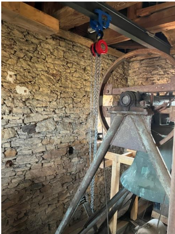
Bilder 1 und 2: Eine Kranbahn wird an der Dachkonstruktion befestigt. Um die Glocke vor Beschädigungen zu schützen, wird sie mit Flies ummantelt.
